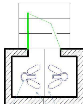
Dalle permettant la séparation urine et excréta Bidon de stockage des urines 2 fosses pour les excréta utilisées alternativement
